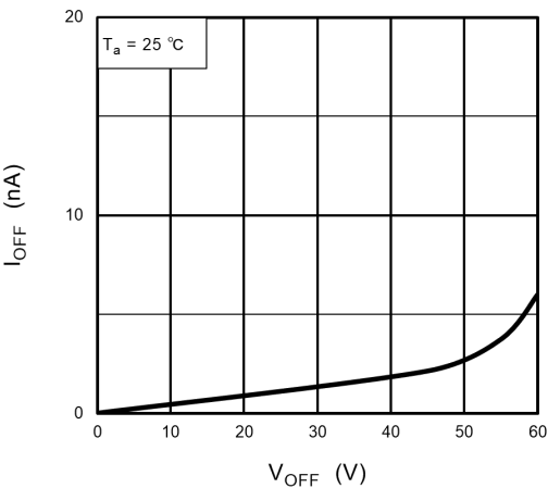
Fig. 12.10 I_{OFF} - V_{OFF}
