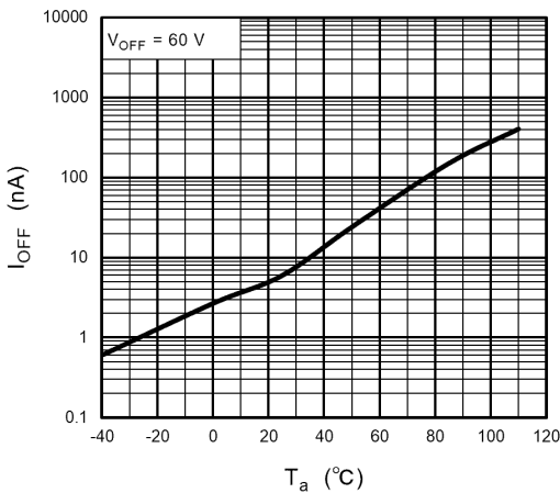
Fig. 12.9 I_{OFF} - T_a
