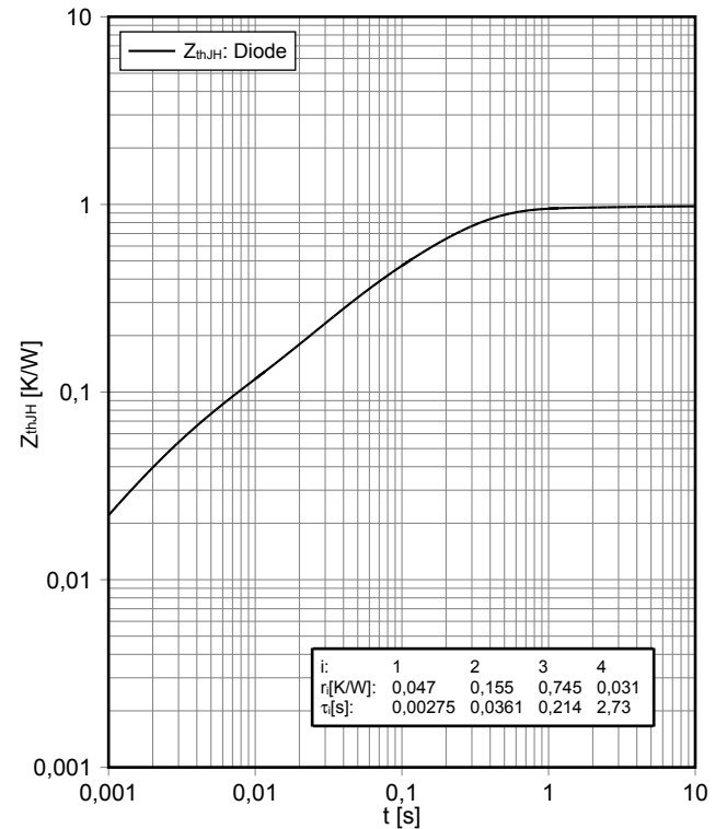
Transienter Wärmewiderstand Diode, Gleichrichter transient thermal impedance Diode, Rectifier Z_{thJH} = f(t)
