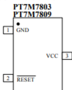
SOT23-3/SC70-3
