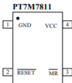
SOT143-4
