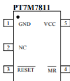
SOT23-5
