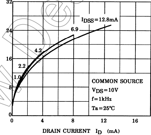
|Y_{fs}| - I_D
