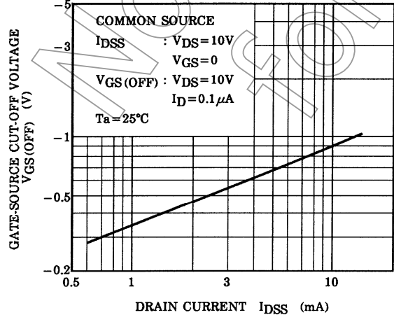
V_{GS}(\text{OFF}) - I_{DSS}
