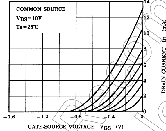
I_D - V_{GS}
