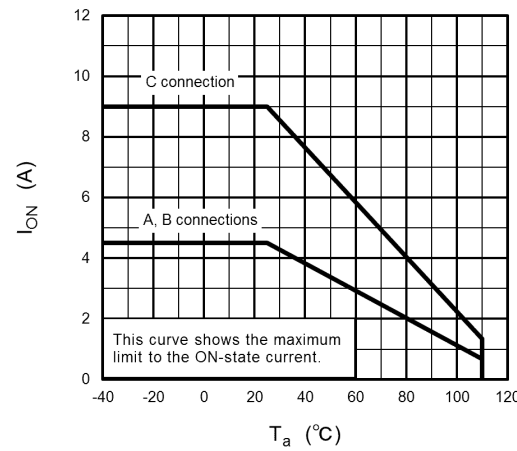
Fig. 12.1.2 I_{ON} - T_a
