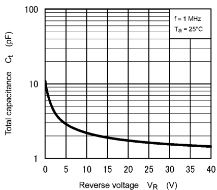
Fig. 9.3 C_t - V_R
