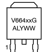
DPAK DT SUFFIX CASE 369C
