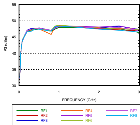
Input IP3
