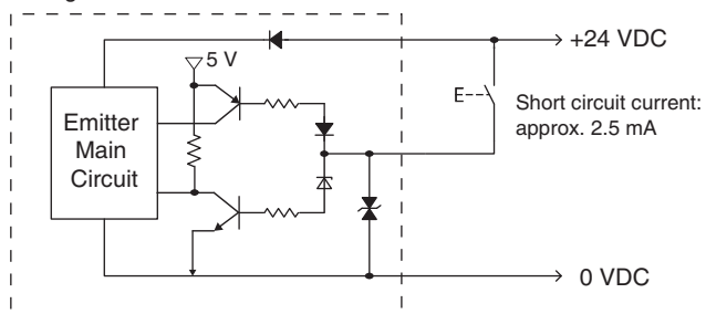
<Long Mode>
