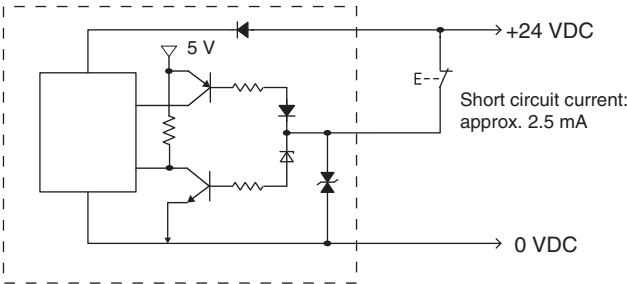
<24 V Inactive>
