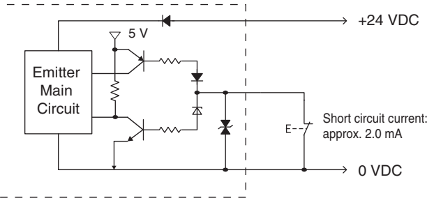
<0 V Inactive>
