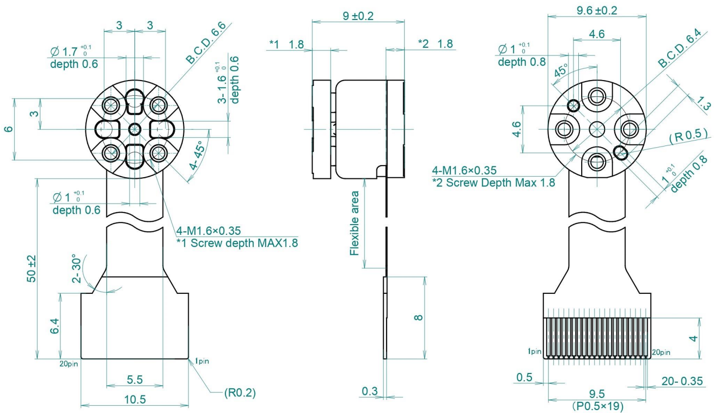
Fig. 27 Dimensions
