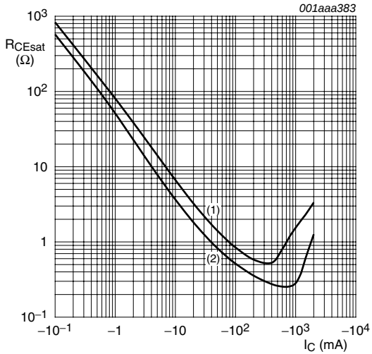
T_{amb} = 25^\circ C (1) I_C/I_B = 50 (2) I_C/I_B = 20
