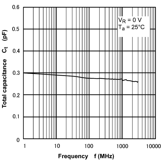
Fig. 9.4 C_t - f
