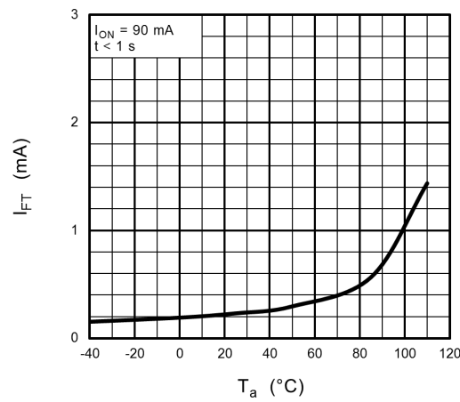
Fig. 14.6 I_{FT} - T_a
