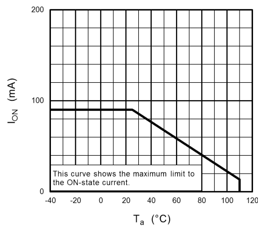
Fig. 14.2 I_{ON} - T_a
