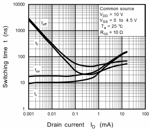
Fig. 9.9 t - I_D
