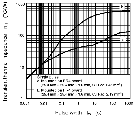
Fig. 9.11 r_{th} - t_w
