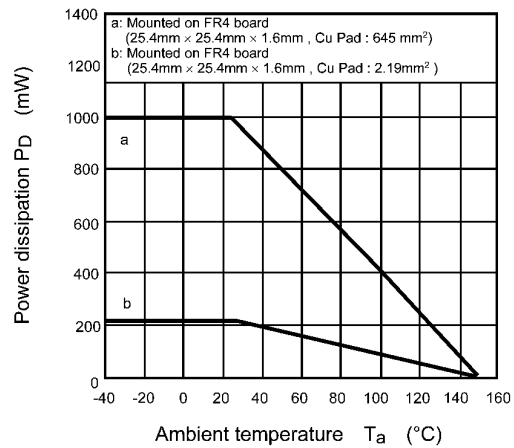
Fig. 9.12 P_D - T_a
