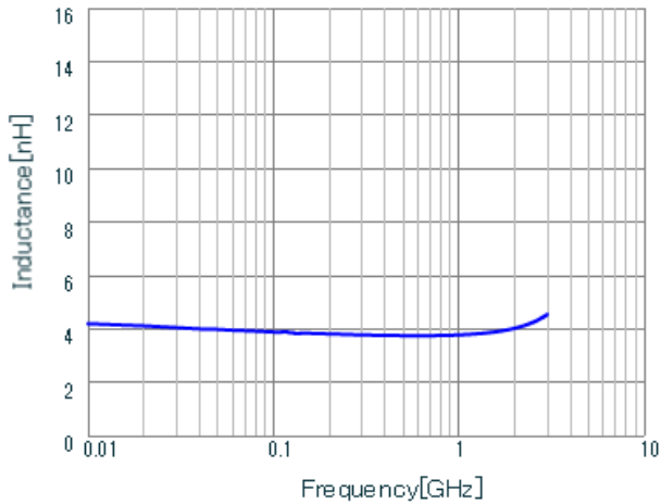
LQG15HN3N9C02 L.
