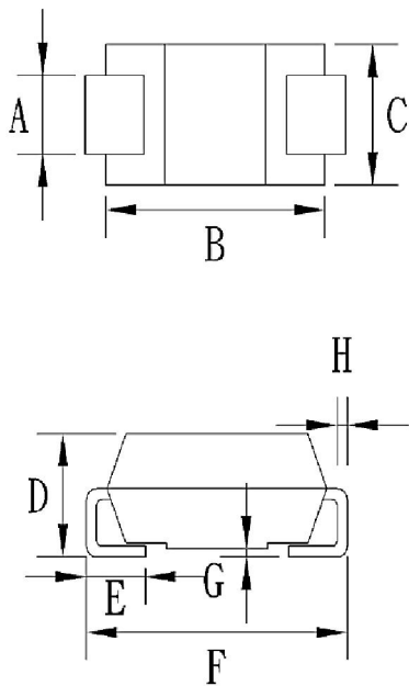
DO-214AC (SMA)
