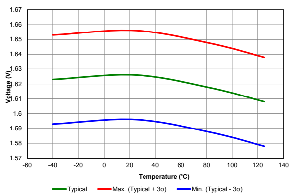
Figure 39-64. POR Release Voltage (VREGPM = 0x)
