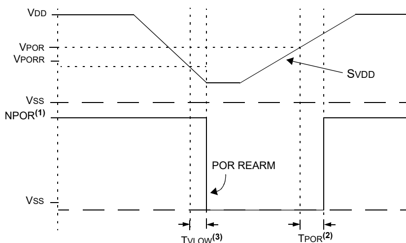
Figure 38-2. POR and POR Rearm with Slow Rising V DD
