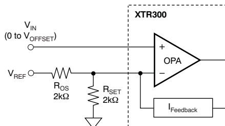
b) Noninverting Input
