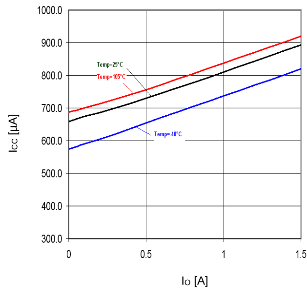
Fig.32 I_o - I_{cc}
