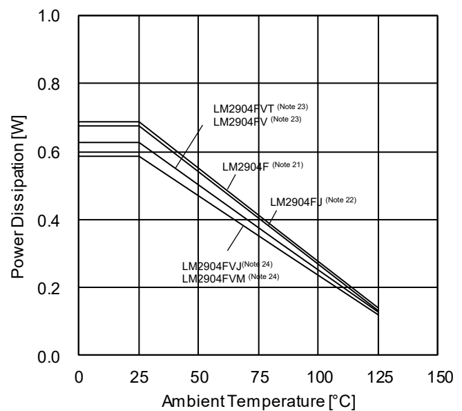
(d) LM2904xxx *2
