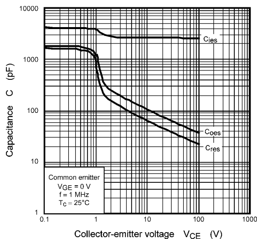
Fig. 8.7 C - V_{CE}
