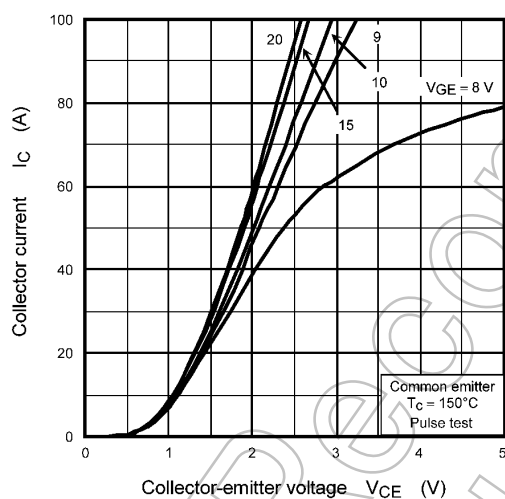
Fig. 8.3 I_C - V_{CE}
