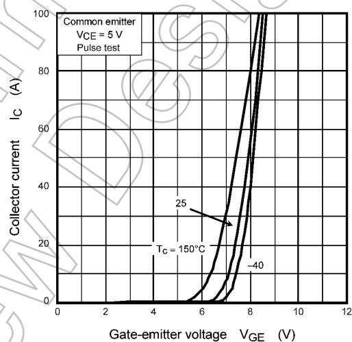
Fig. 8.4 I_C - V_{GE}
