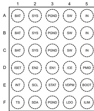
bq24250 DSBGA
