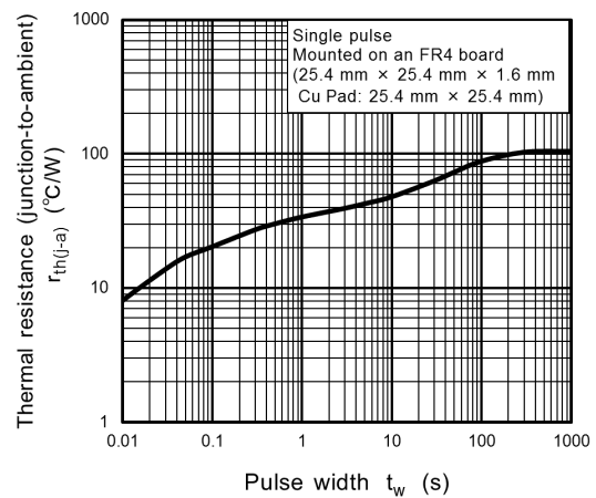
Fig. 9.4 r_{th} - t_w
