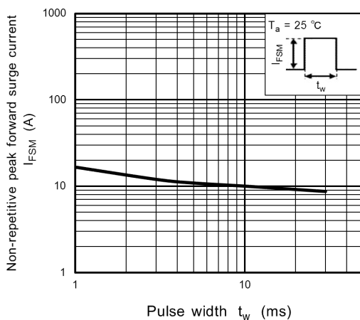
Fig. 9.5 I_{FSM} - t_w
