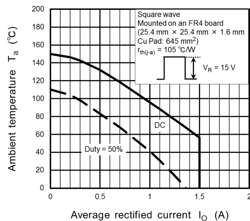
Fig. 9.6 T_a - I_O
