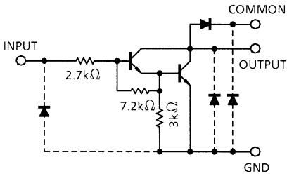
TD62003APG/AFG
