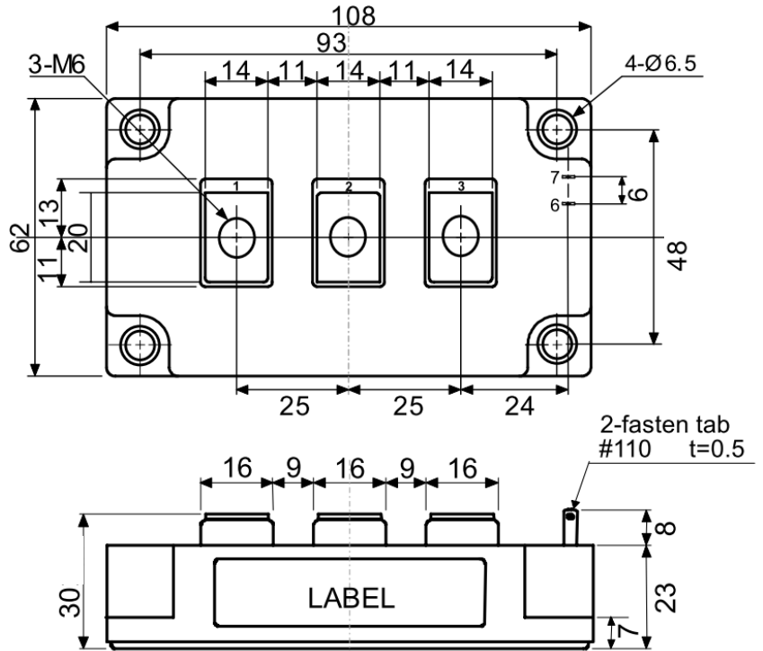
□ 概略図 : SCHEMATIC DIAGRAM
