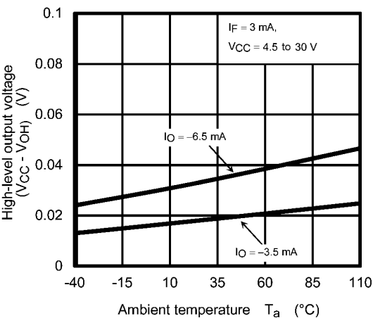
Fig. 12.2.6 (V_{CC} - V_{OH}) - T_a
