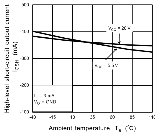
Fig. 12.2.10 I_{osH} - T_a
