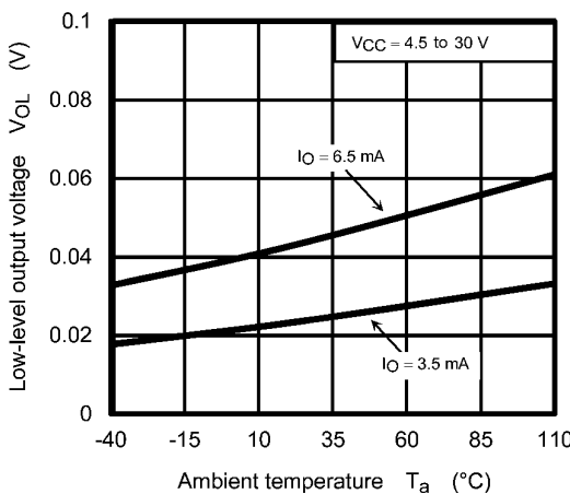
Fig. 12.2.5 V_{OL} - T_a
