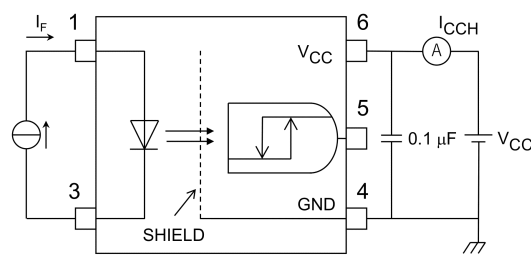
Fig. 12.1.4 I_{CCH} Test Circuit
