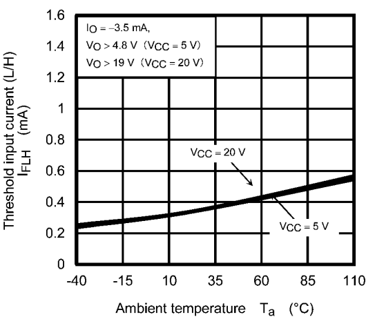
Fig. 12.2.2 I_{FLH} - T_a
