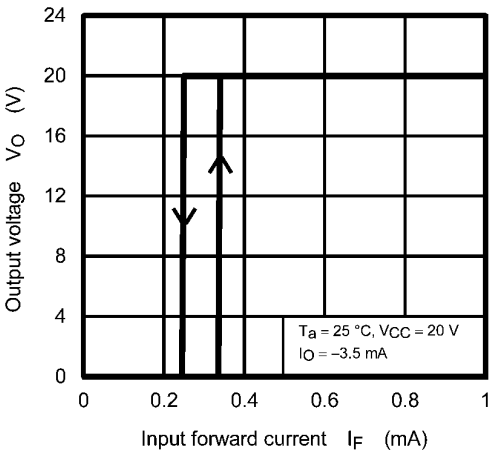
Fig. 12.2.4 V_O - I_F (I_{HYS})
