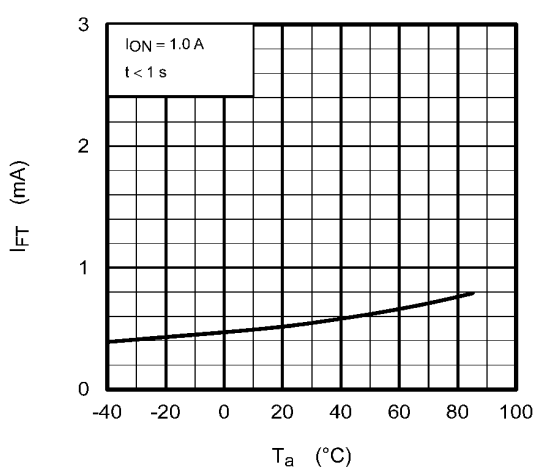
Fig. 16.6 I FT - T a
