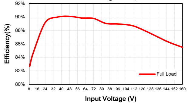
EC7BW18-72D24 Eff Vs Vin @25 Deg. C
