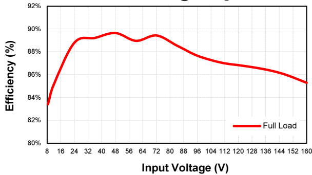
EC7BW18-72D15 Eff Vs Vin @25 Deg. C
