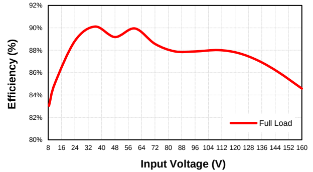
EC7BW18-72D12 Eff Vs Vin @25 Deg. C
