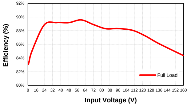
EC7BW18-72S15 Eff Vs Vin @25 Deg. C
