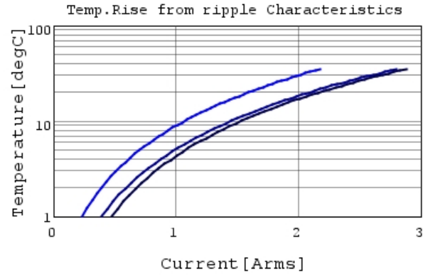
GCJ188C70J335KE02 Temp.rise — 100kHz
