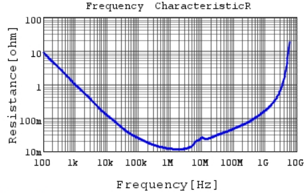
GCJ188C70J335KE02 R DCOV, 25degC
