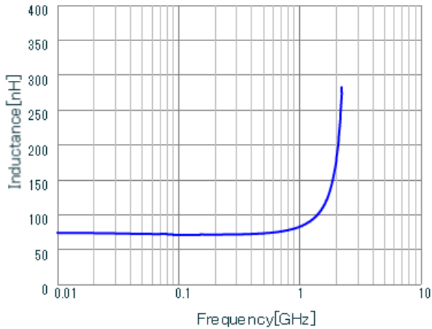
LQW18AN72NG00 L.
