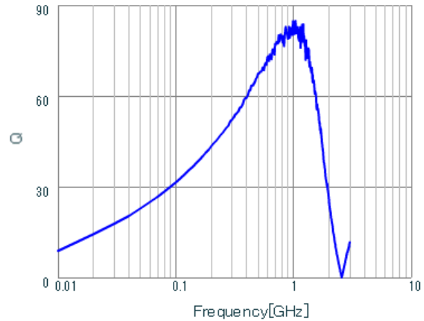
LQW18AN72NG00 Q.
