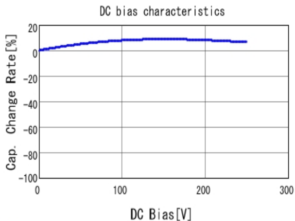
■ DE2E3KY102MN3AM02F C-DC bias capchange, 20.0degC, AC1
