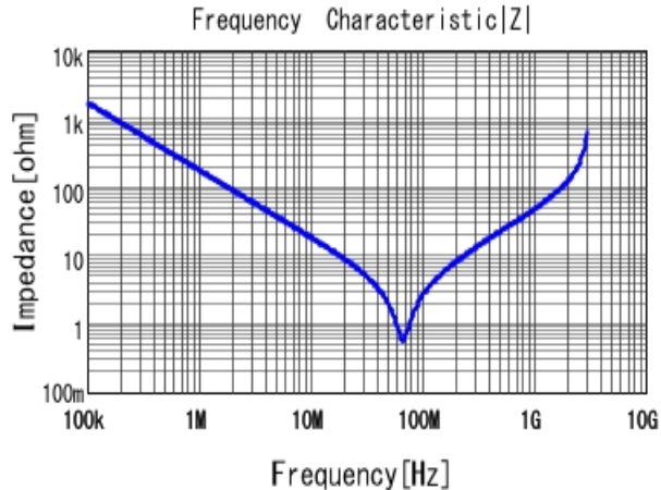
■ DE2E3KY102MN3AM02F |Z| DCOV, 20degC
