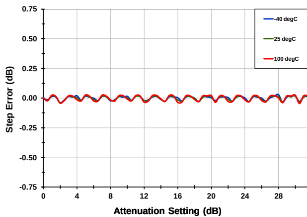
DNL [2800 MHz]
