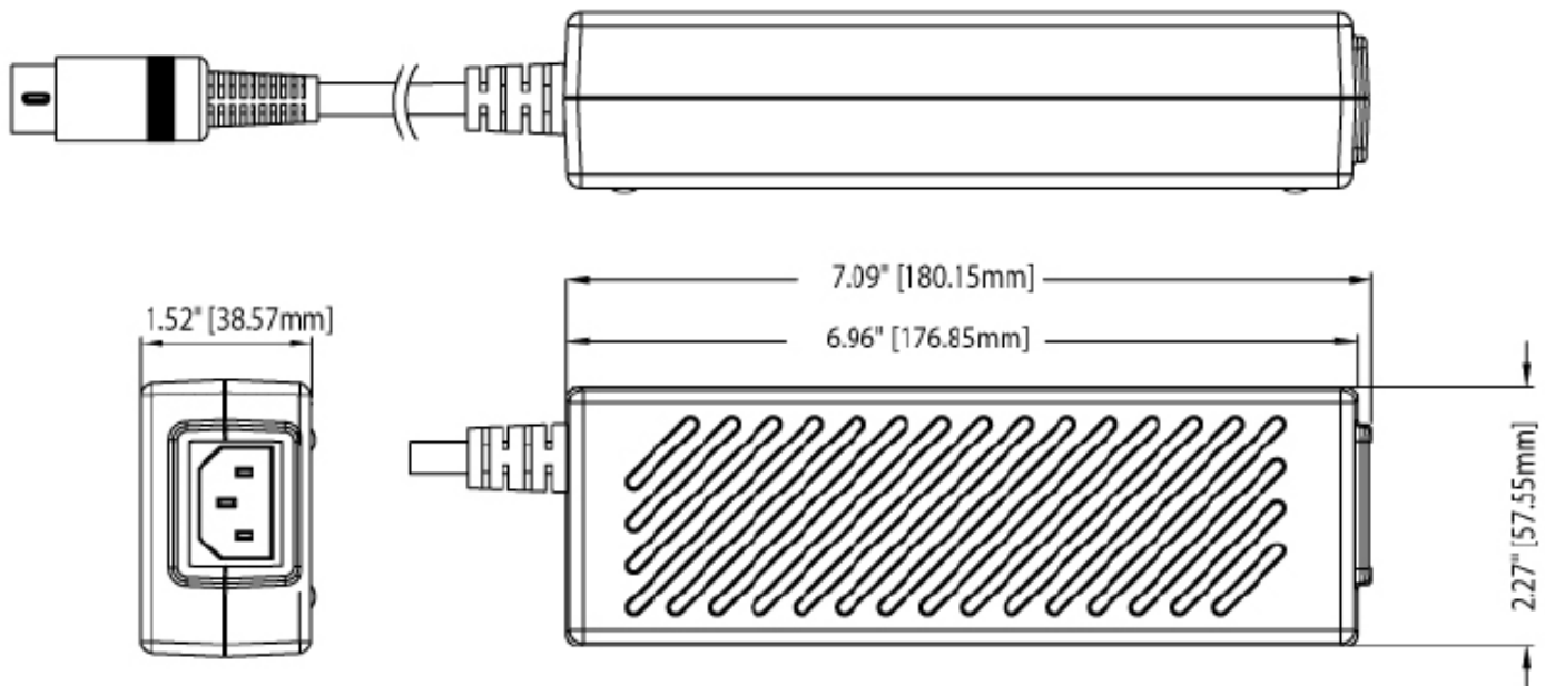
MWC100-DWG
