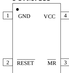
SOT143-4
