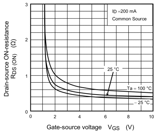
Fig. 7.3 R_{DS(ON)} - V_{GS}
