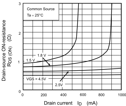
Fig. 7.4 R_{DS(ON)} - I_D
