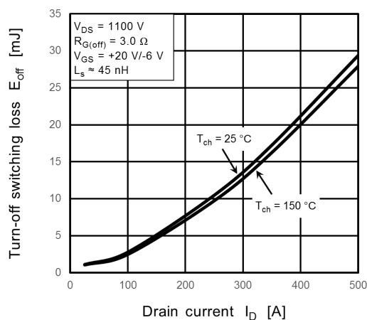
Fig. 8.8 E_{off} - I_D
