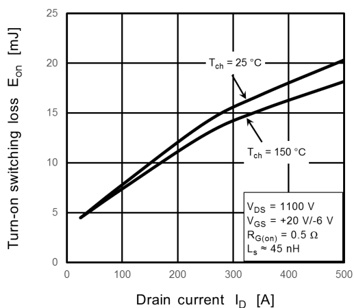
Fig. 8.7 E_{on} - I_D
