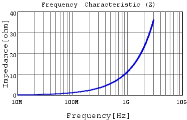
LQW18AS1N8J0Z |Z|
