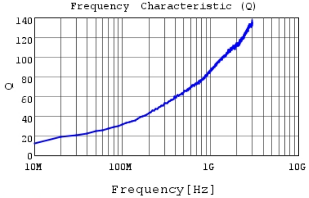
LQW18AS1N8J0Z Q
