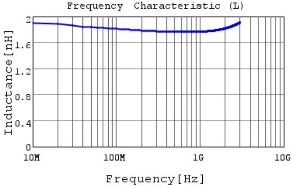
LQW18AS1N8J0Z L
