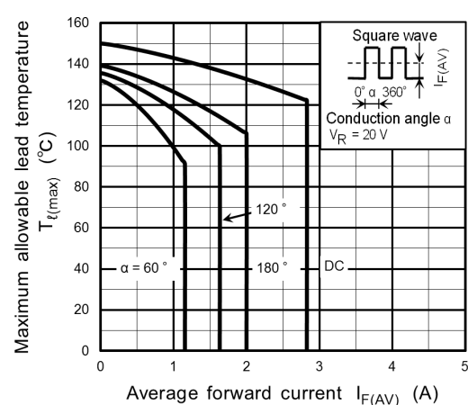
Fig. 10.4 T_{l(max)} - I_{F(AV)}
