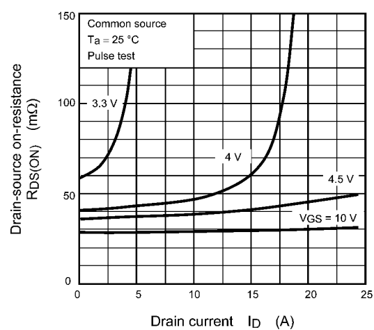
Fig. 9.4 R_{DS(ON)} - I_D
