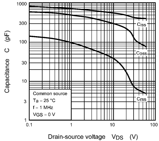
Fig. 9.8 C - V_{DS}
