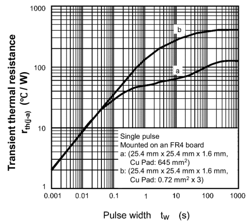
Fig. 9.12 r_{th(j-a)} - t_w
