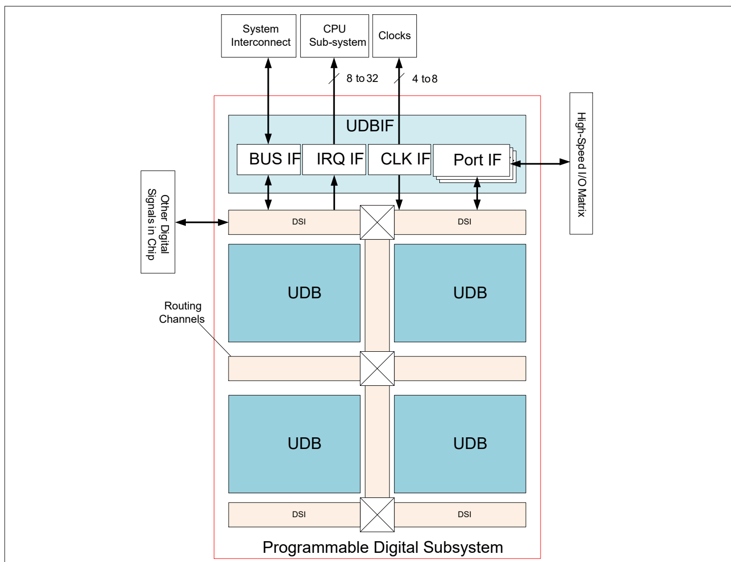
Figure 4 UDB array
