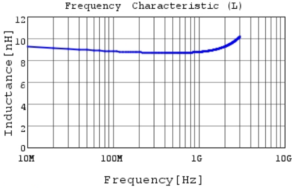
LQW18AN8N7D00 L
