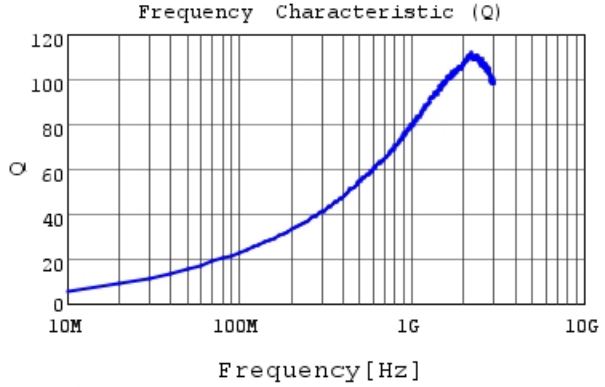
LQW18AN8N7D00 Q
