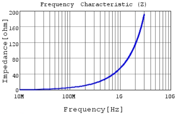
LQW18AN8N7D00 |Z|
