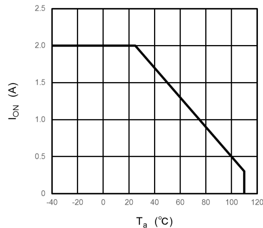
Fig. 14.2 I_{ON} - T_a
