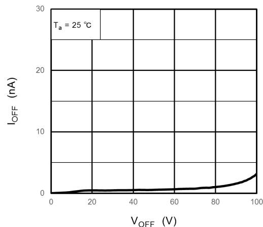
Fig. 14.10 I_{OFF} - V_{OFF}
