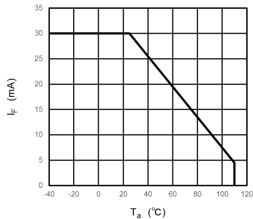
Fig. 14.1 I_F - T_a
