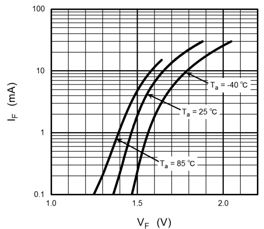
Fig. 14.3 I_F - V_F
