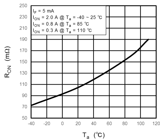
Fig. 14.5 R_{ON} - T_a
