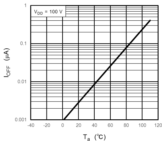
Fig. 14.9 I_{OFF} - T_a
