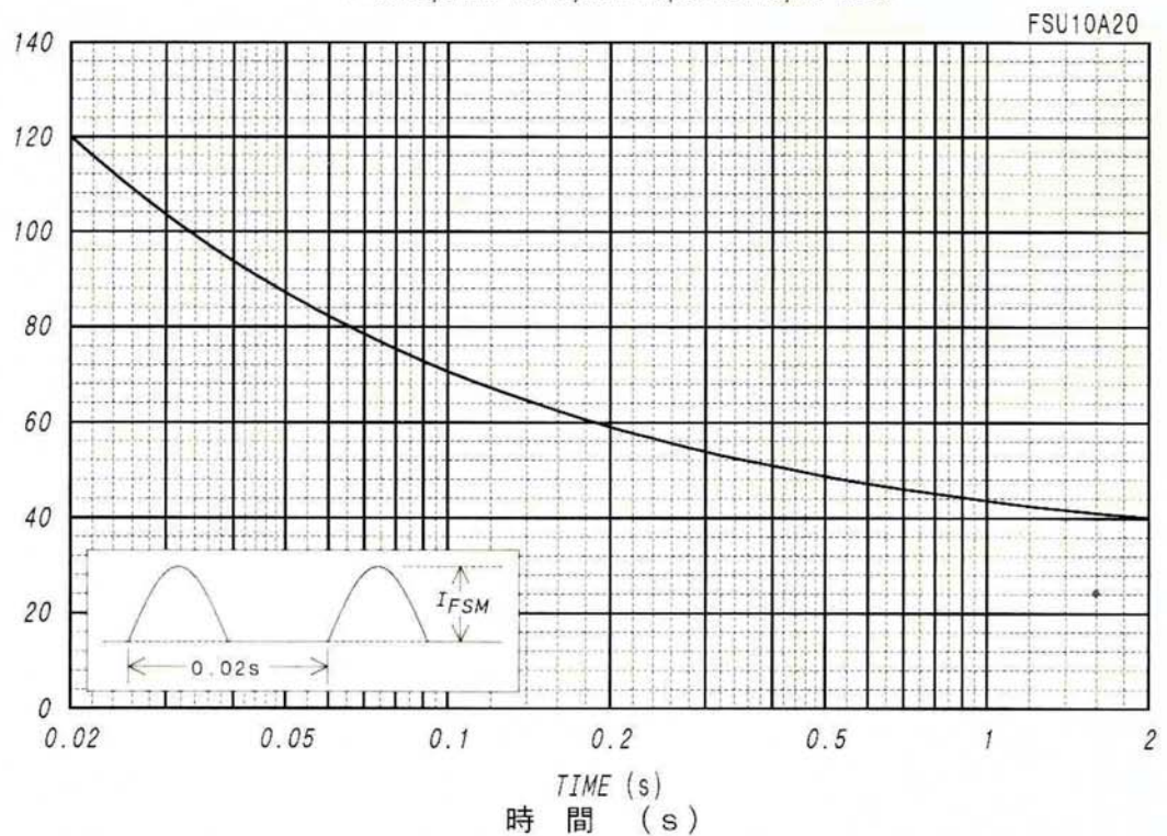
サージ順電流定格 SURGE CURRENT RATINGS
