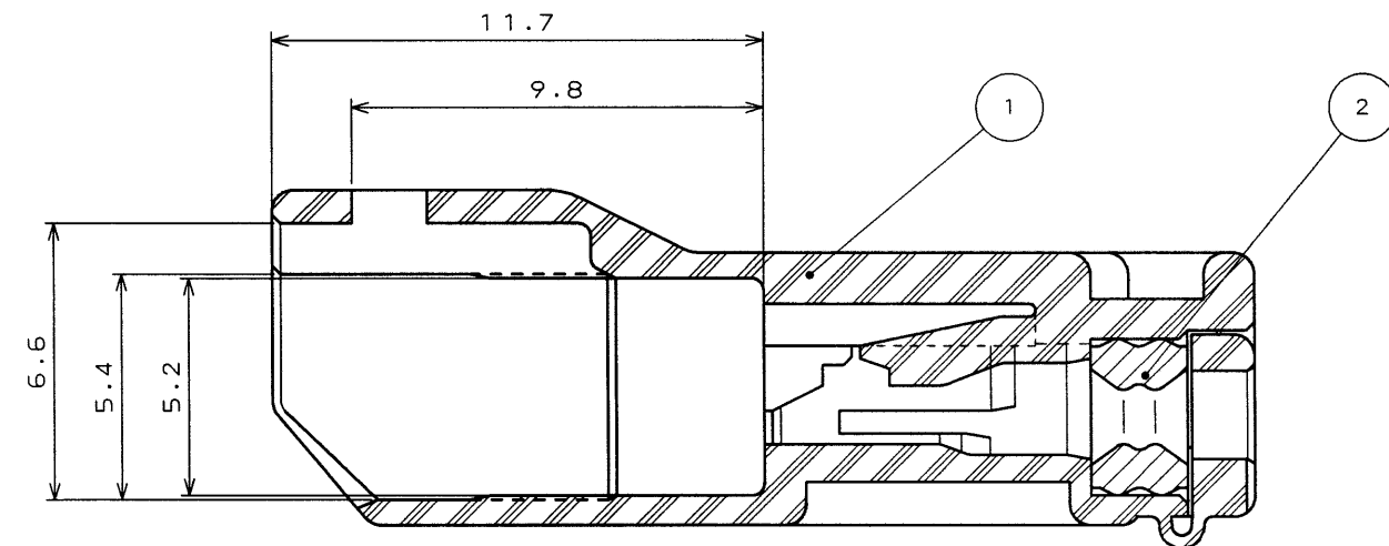
SECT. A-A (SCALE 5:1)
