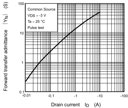
Fig. 9.8 |Y_{fs}| - I_D
