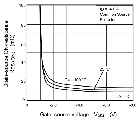
Fig. 9.4 R_{DS(ON)} - V_{GS}
