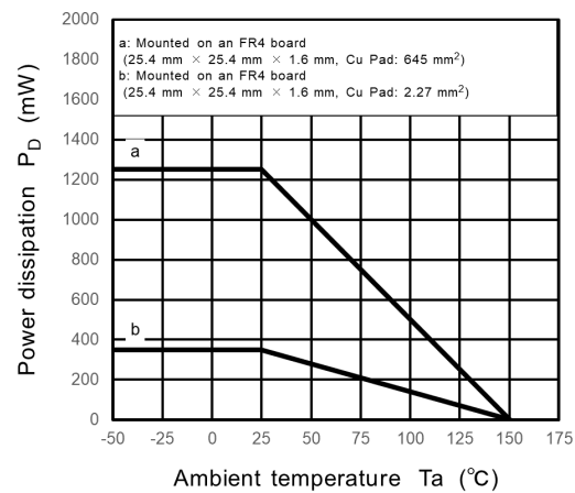
Fig. 9.14 P_D - T_a
