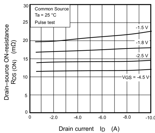
Fig. 9.5 R_{DS(ON)} - I_D
