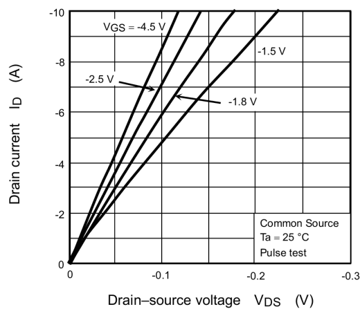
Fig. 9.1 I_D - V_{DS}
