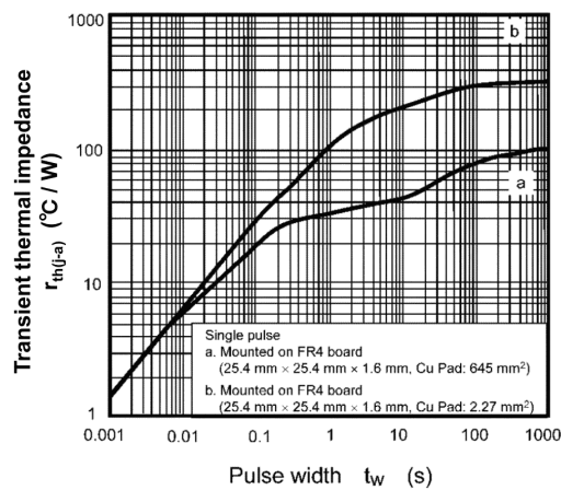
Fig. 9.13 r_{th(j-a)} - t_w
