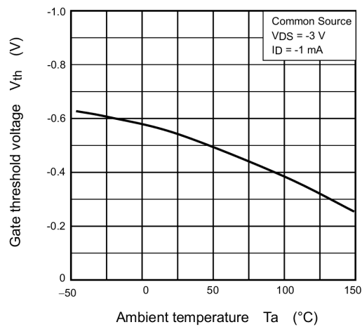
Fig. 9.7 V_{th} - T_a
