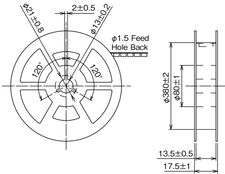
Reel Dimensions
