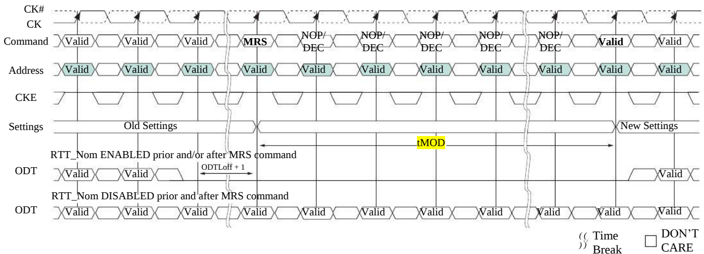
Figure 2.3.1b tMOD Timing
