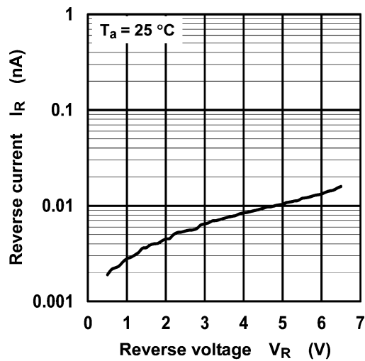
Fig. 8.2 I_R - V_R
