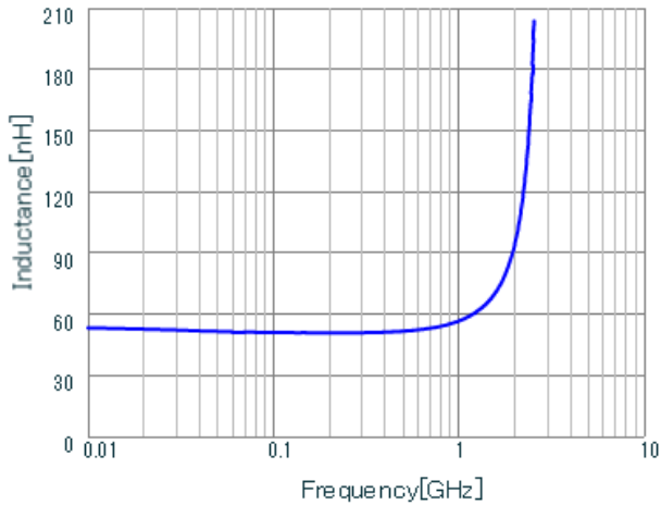
LQW18AN51NJ00 L.
