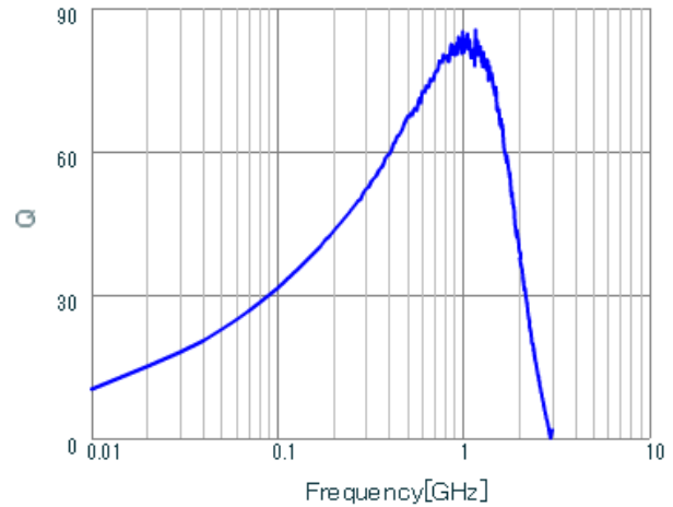
LQW18AN51NJ00 Q.
