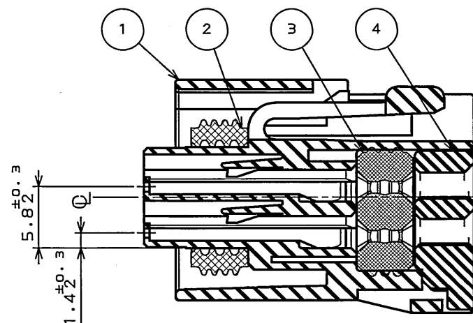
SECT. A-A (SCALE 2:1)
